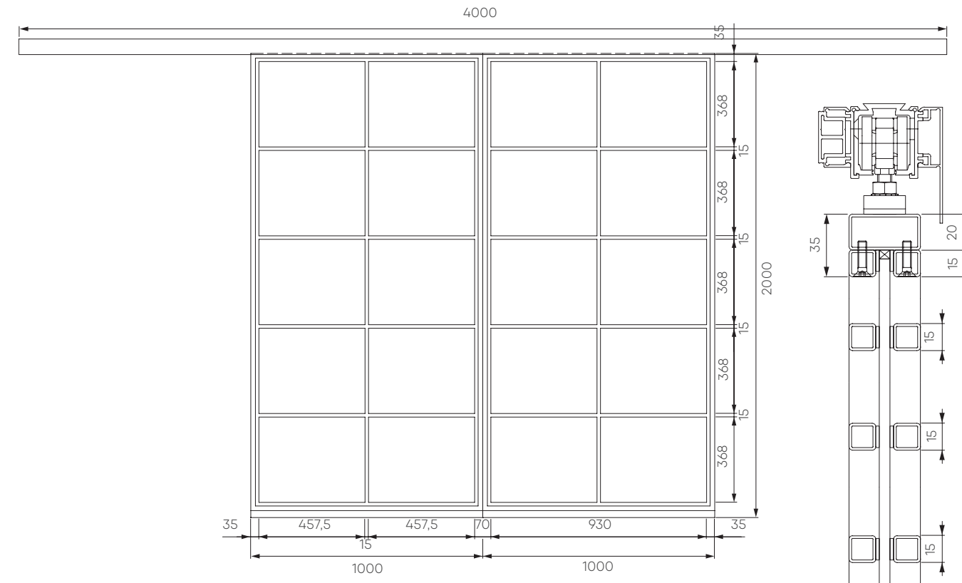
2-flügelige Stahl-Loft-Schiebetür
