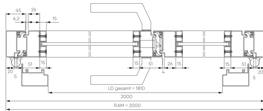
Horizontalschnitt 2-flügelige Stahl-Lofttür
