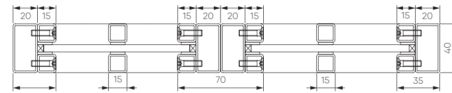
2-flügelige Stahl-Loft-Schiebetür
