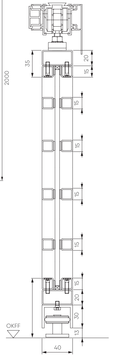
Vertikalschnitt 2-flügelige Stahl-Loft-Schiebetür
