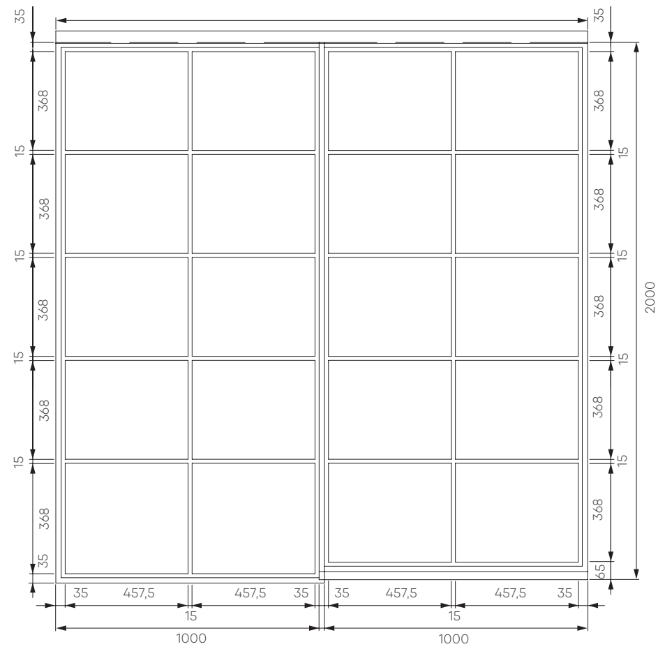
1-flügelige Stahl-Loft-Schiebetür mit Seitenteil
