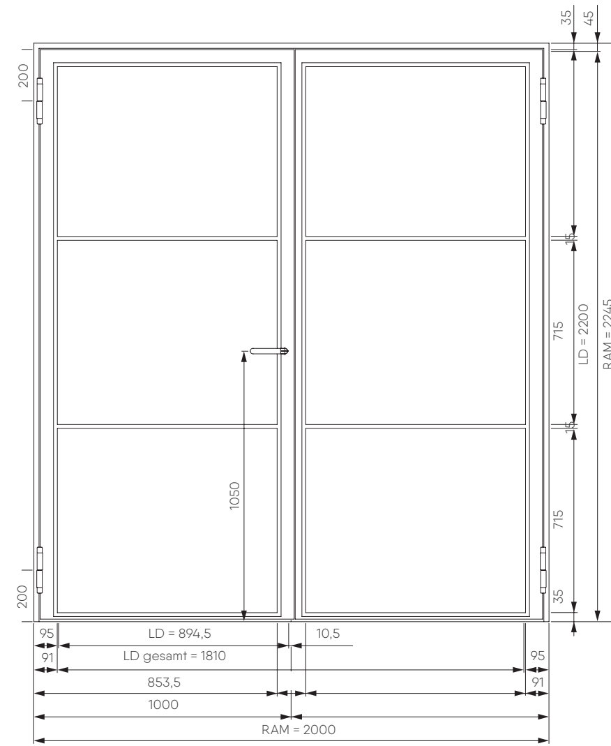
2-flügelige Stahl-Lofttür
