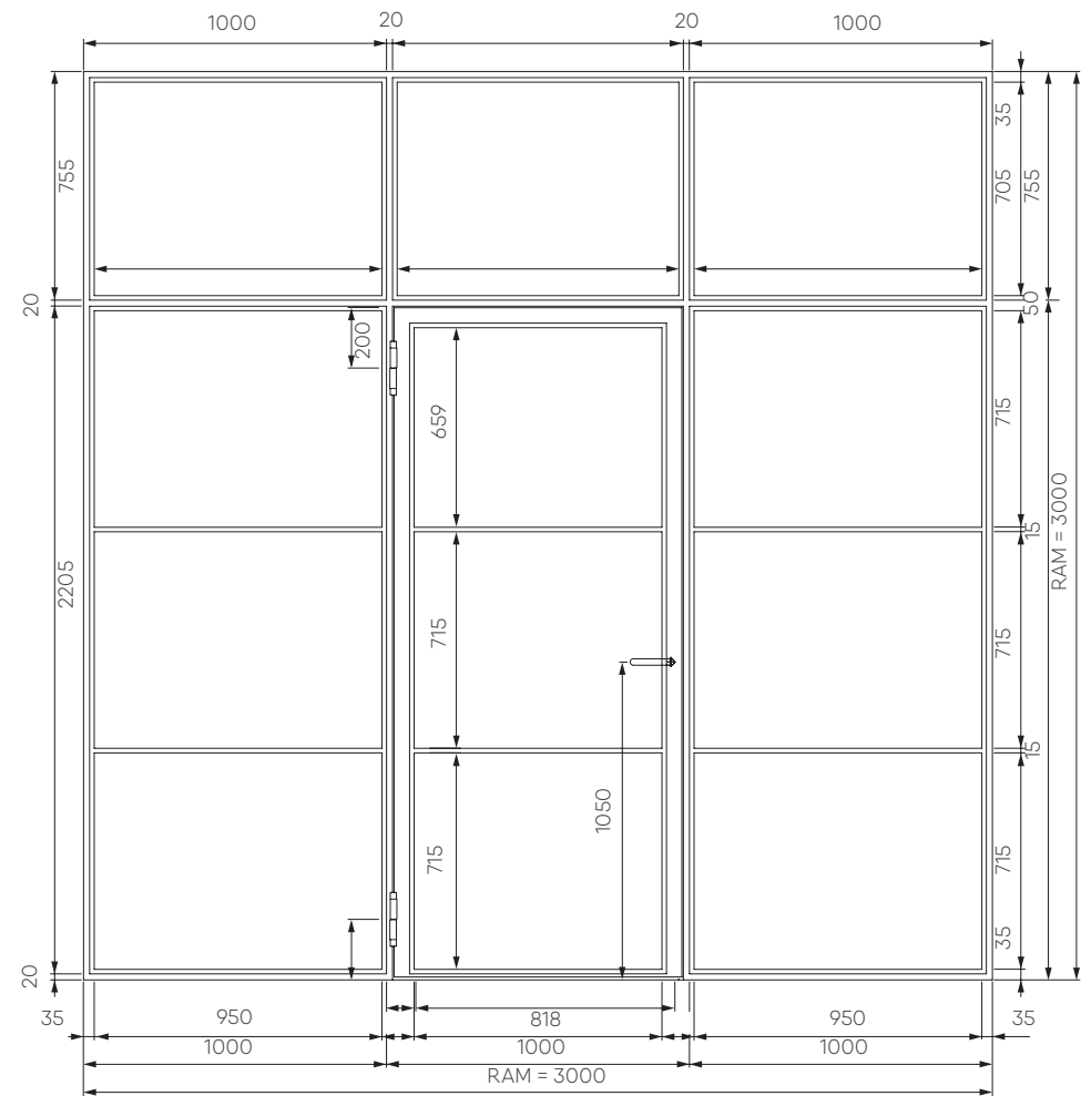
1-flügelige Stahl-Lofttür mit Seitenteilen und Oberlicht
