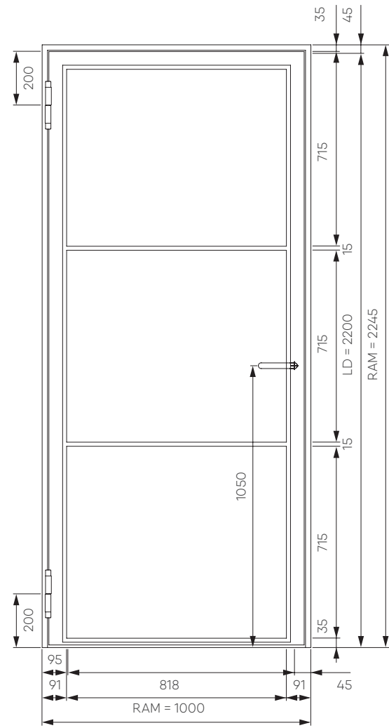
1-flügelige Stahl-Lofttür
