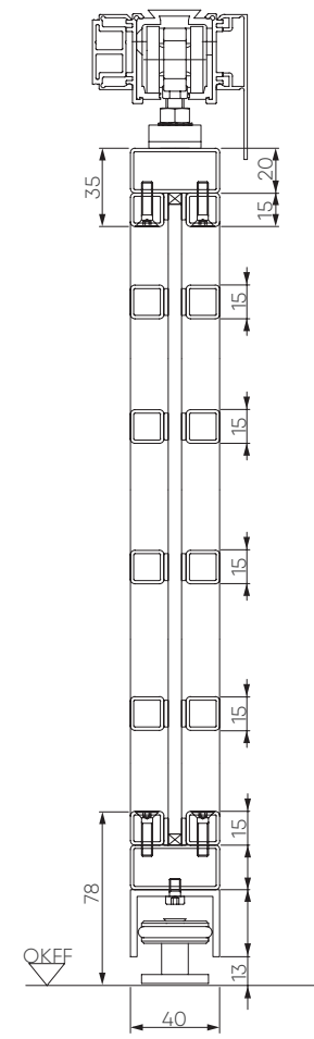
Vertikalschnitt 1-flügelige Stahl-Loft-Schiebetür
