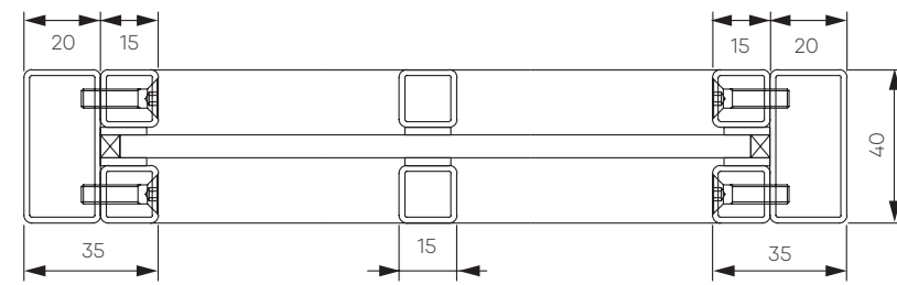
Horizontalschnitt 1-flügelige Stahl-Loft-Schiebetür
