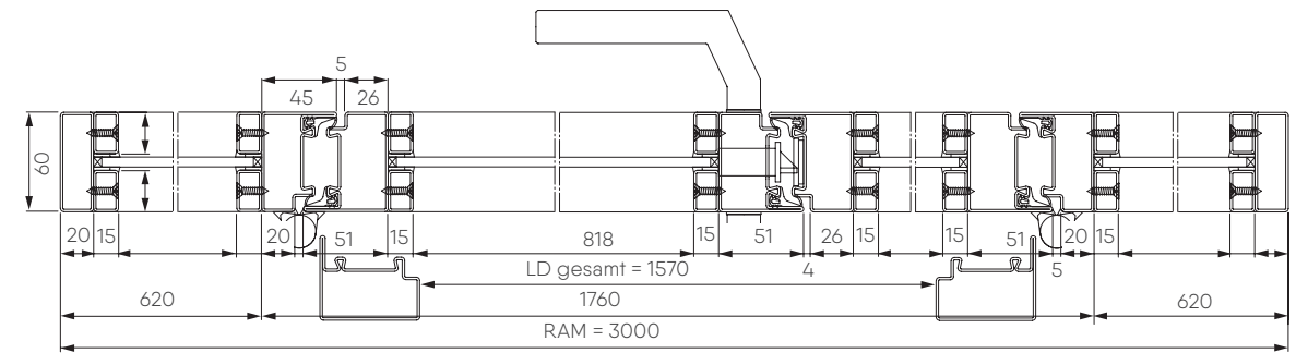
Horizontalschnitt 2-flügelige Stahl-Lofttür mit Seitenteilen
