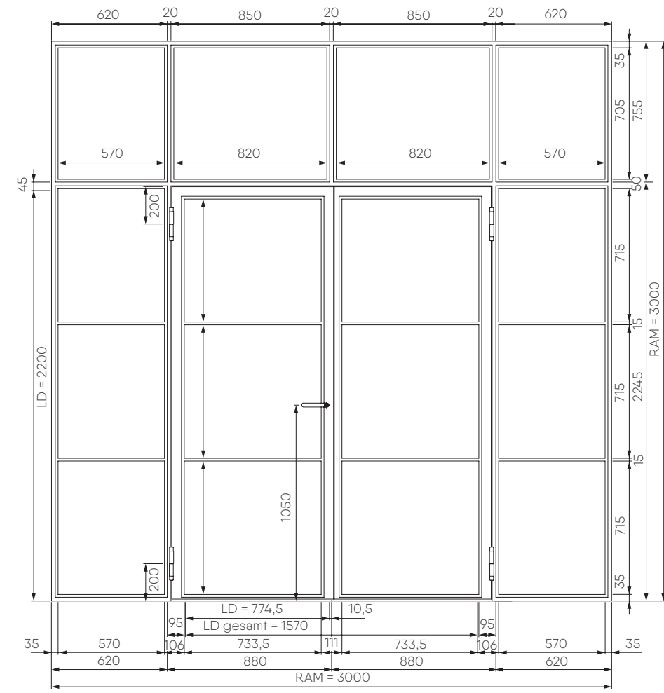
2-flügelige Stahl-Lofttür mit Seitenteilen und Oberlicht
