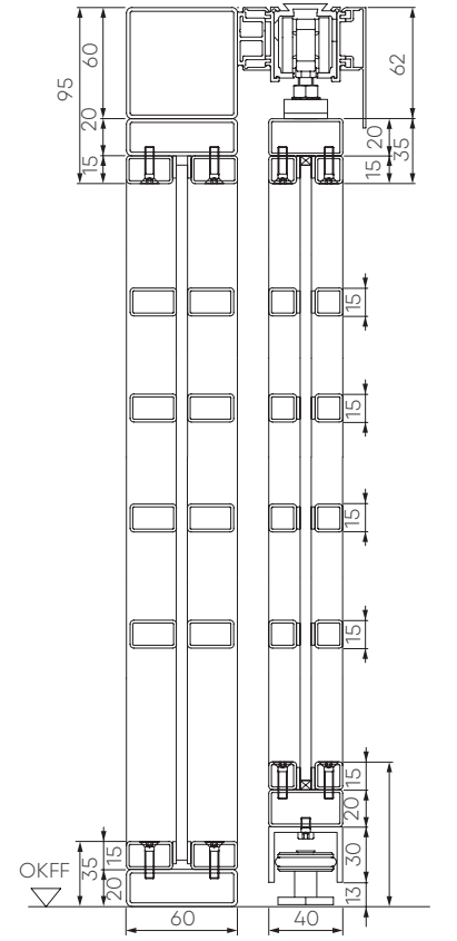
Vertikalschnitt 2-flügelige Stahl-Loft-Schiebetür mit Seitenteil
