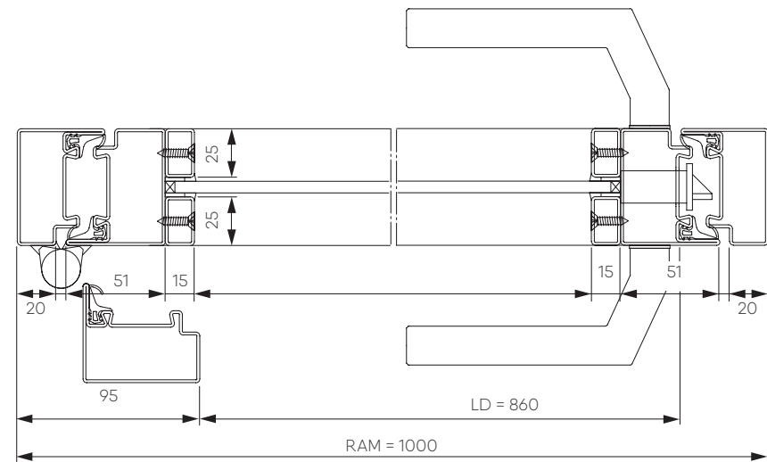
1-flügelige Stahl-Lofttür
