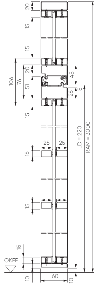
Vertikalschnitt 2-flügelige Stahl-Lofttür mit Oberlicht
