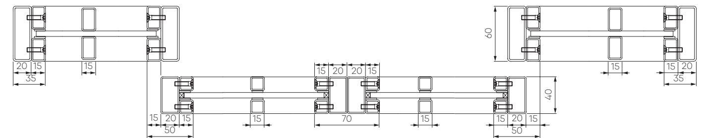
Horizontalschnitt 2-flügelige Stahl-Loft-Schiebetür mit Seitenteil
