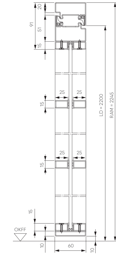
Vertikalschnitt 1-flügelige Stahl-Lofttür
