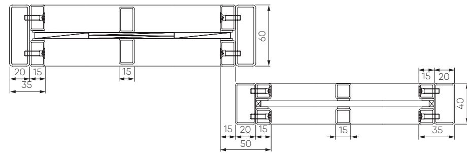
Horizontalschnitt 1-flügelige Stahl-Loft-Schiebetür mit Seitenteil
