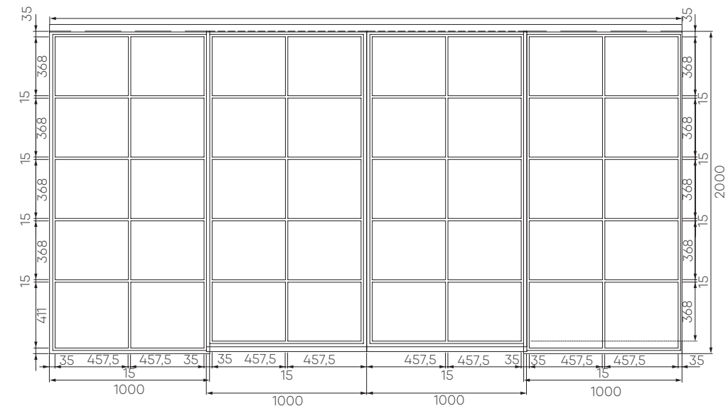
2-flügelige Stahl-Loft-Schiebetür mit Seitenteil
