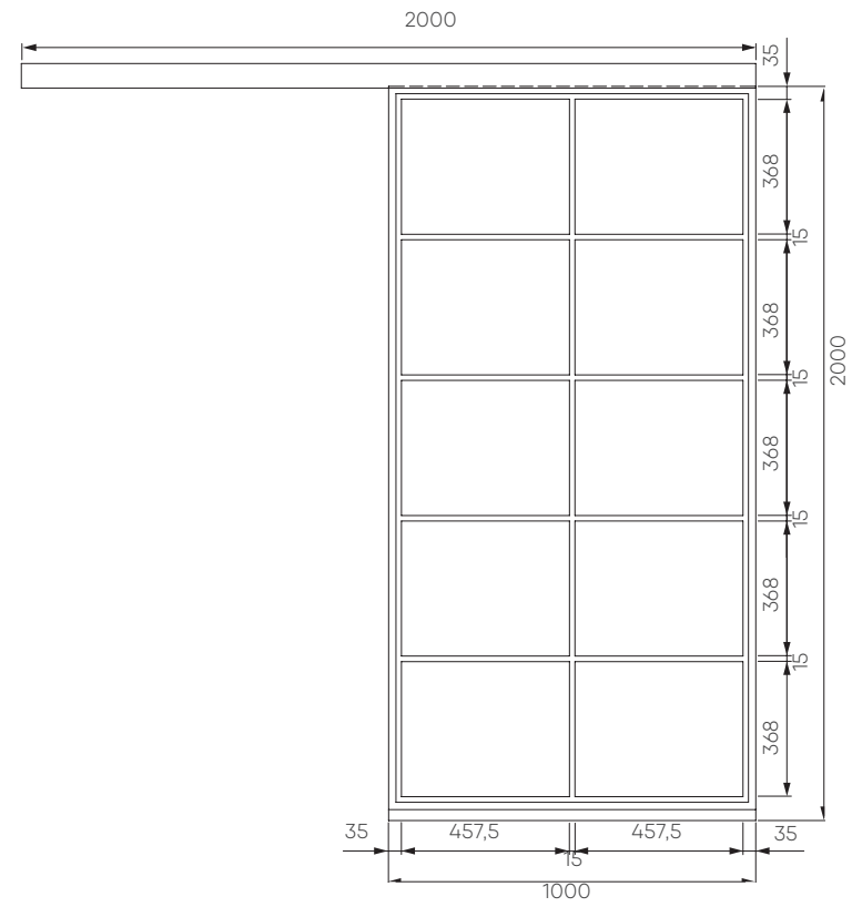
1-flügelige Stahl-Loft-Schiebetür
