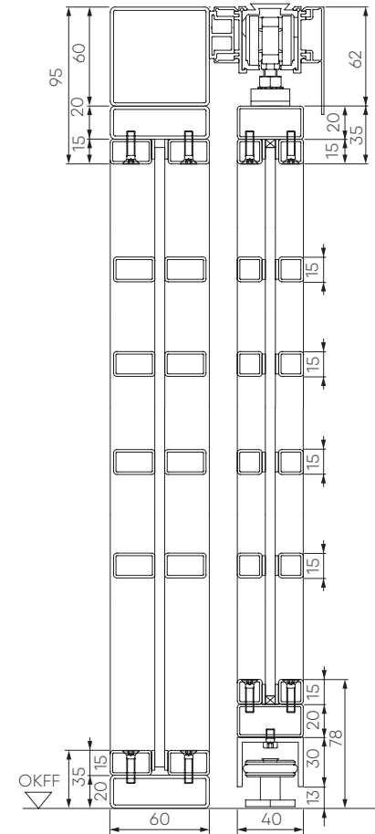
Vertikalschnitt 1-flügelige Stahl-Loft-Schiebetür mit Seitenteil
