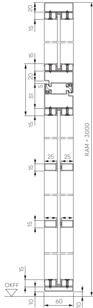
Vertikalschnitt 1-flügelige Stahl-Lofttür mit Oberlicht
