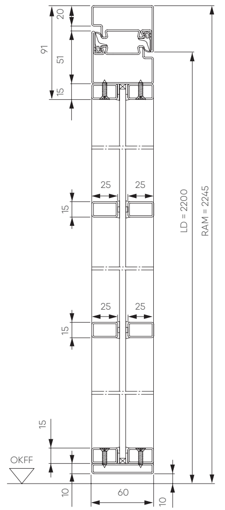
Vertikalschnitt 2-flügelige Stahl-Lofttür
