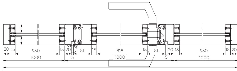
Horizontalschnitt 1-flügelige Stahl-Lofttür mit Seitenteilen
